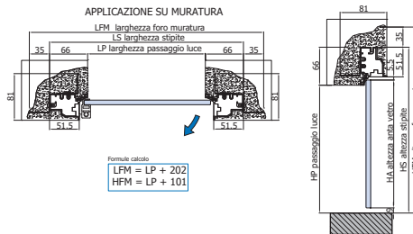
A-Links nach aussen öffnend A-left opening to pull
