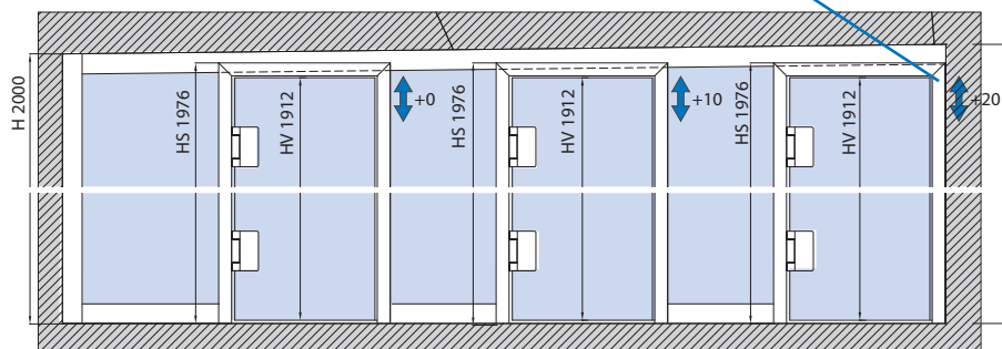
Beispiel optional Verstellung Türzarge mit Trennwandprofil oben Example optional adjustment door frame with top partition profile
