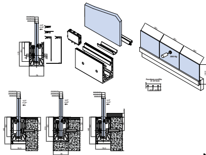
B-6250-G Abdeckungen nicht enthalten Cover profiles not included
